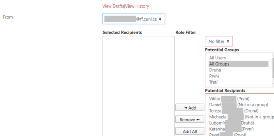
Obr. 6: výběr adresátů
